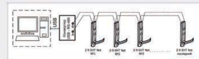
Рис. 1 Схема работы замков Z-9 ENT в сети
