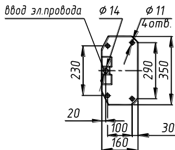
Установочные размеры турникета "Ростов-Дон Т2М1"
