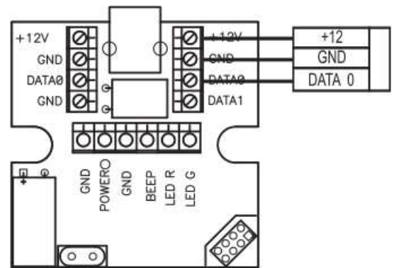
4. Подключение считывателя по Dallas Touch Memory (Ibutton)
