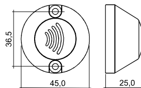
Рис.1 Габариты изделия
