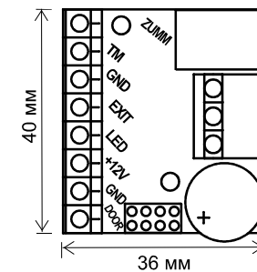
Рис.2 Внешний вид платы.
