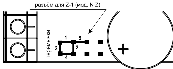
Рис.3 Положение переключек.
