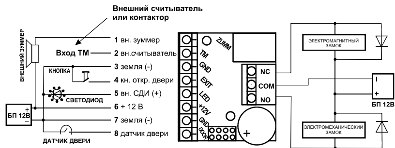
Рис.6 Подключение внешних устройств.
