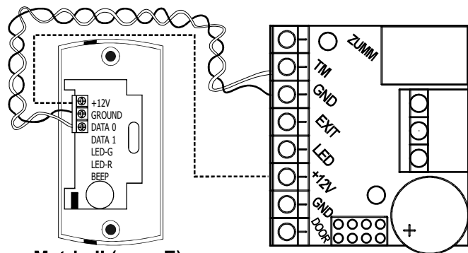
Рис.4 Подключение внешнего считывателя.
