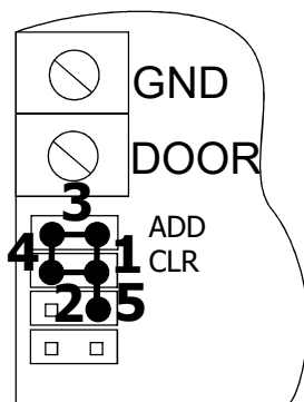
Рис.6 Положения переключки
