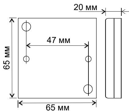
Рис.7 Внешний вид корпуса и габаритные размеры
