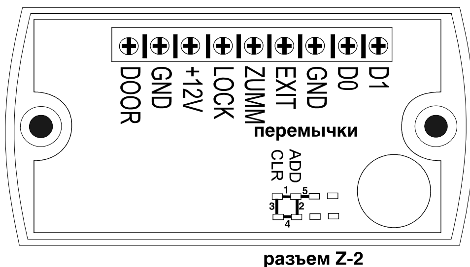
Рис. 3 Положение перемычек
