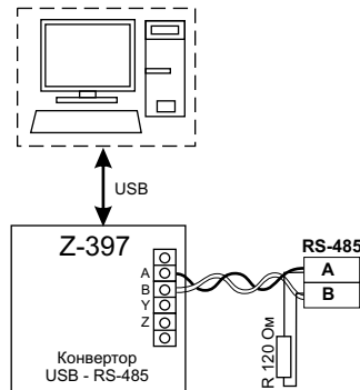
Рис.3 Схема подключения по RS-485
