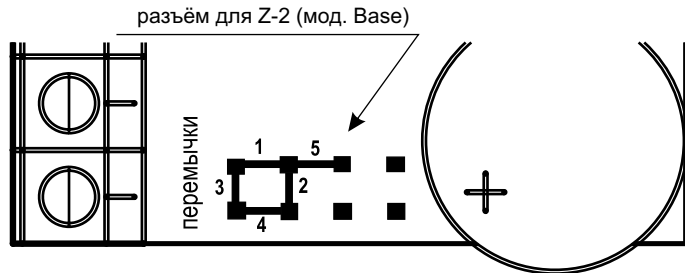
Рис. 3 Положение перемычек
