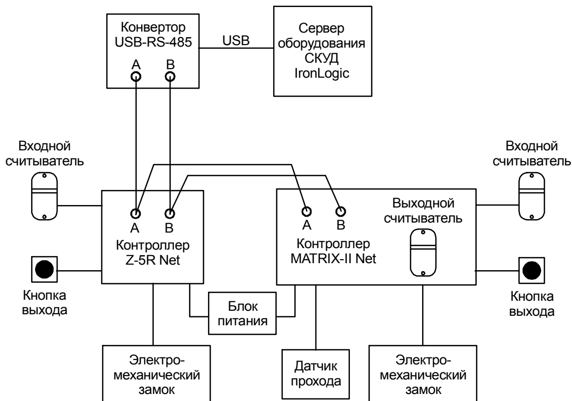
Рисунок 37 – Схема подключения для двух точек прохода
