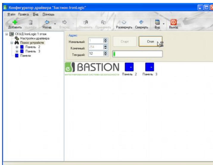
Рисунок 42 – Поиск контроллеров
