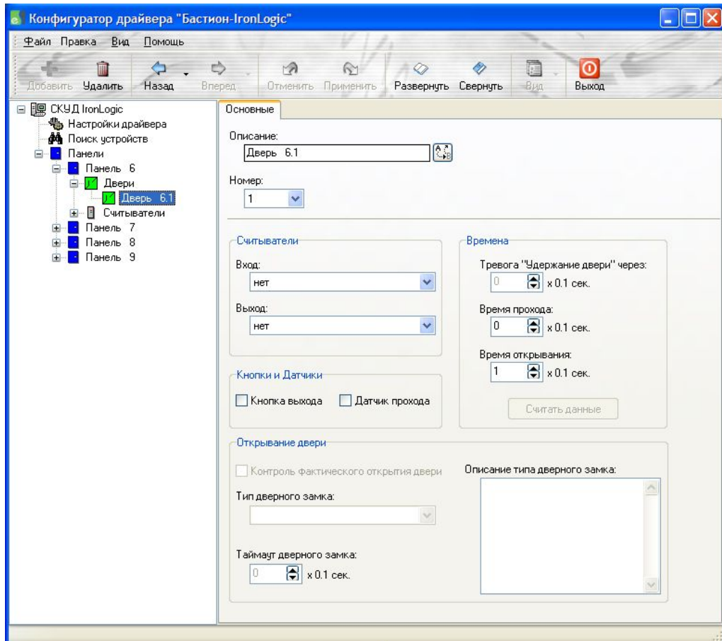
Рисунок 22 – Параметры двери
