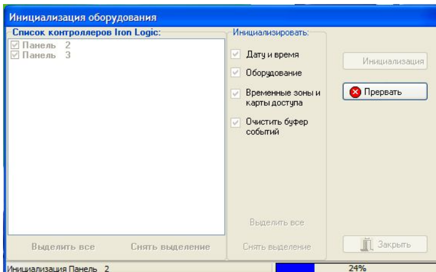
Рисунок 55 – Процесс инициализации
