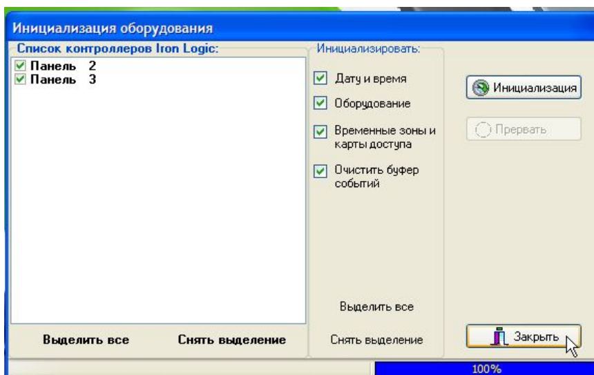
Рисунок 56 – Завершение инициализации
