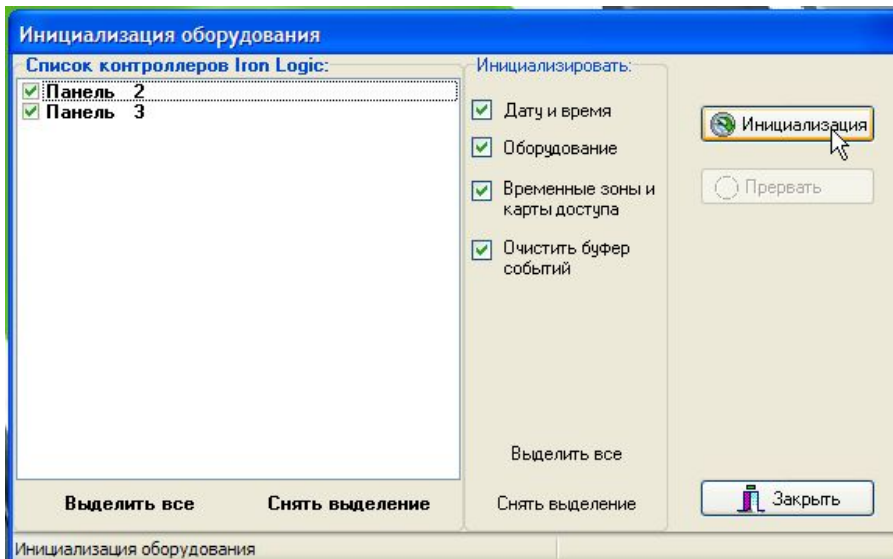
Рисунок 54 – Запуск инициализации
