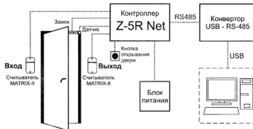
Рисунок 1 – Вариант подключения Z-5R Net
