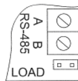
Рисунок 3 - Переключатель LOAD на колодке №2
