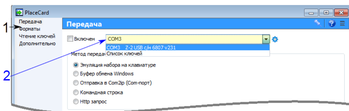
Рисунок 2. Выбор считывателя
