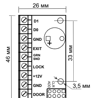
Рис.2 Внешний вид платы контроллера
