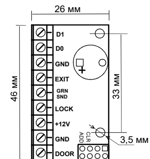
Рис.2 Внешний вид платы контроллера
