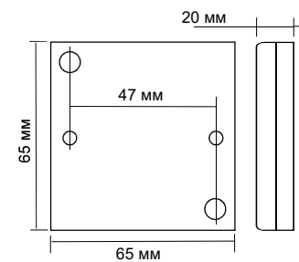
Рис.1 Габаритные размеры корпуса контроллера
