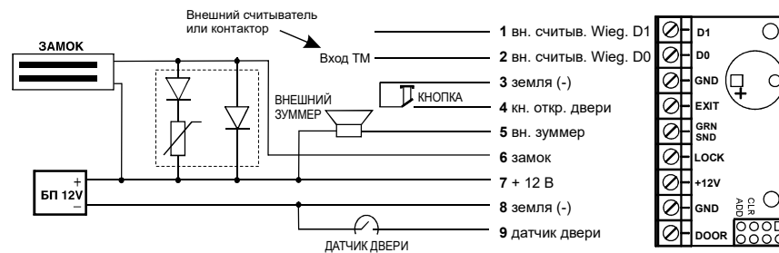
Рис.6 Схема подключения внешних устройств
