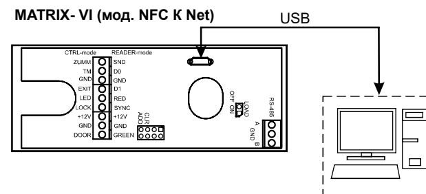
Рис.3 Подключение устройства по USB.
