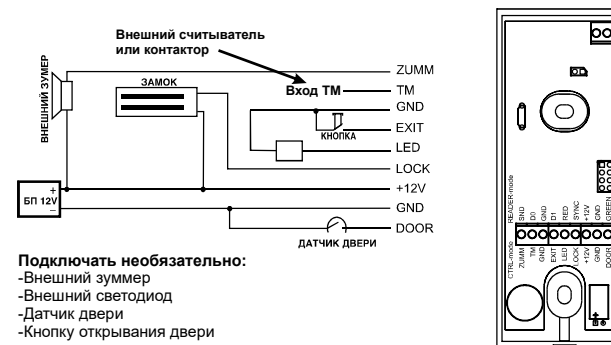
Рис.8 Подключение внешних устройств к контроллеру.
