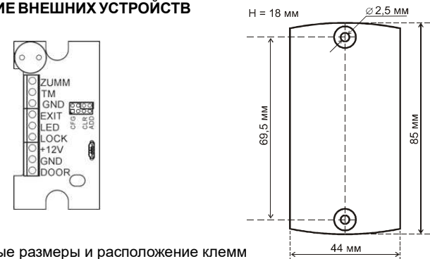
Рис.1 Габаритные размеры и расположение клемм
