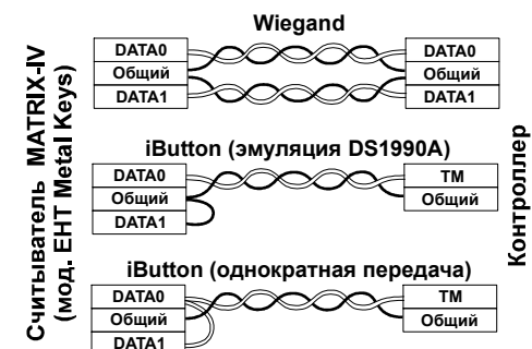
Рис.2 Выбор протокола передачи
