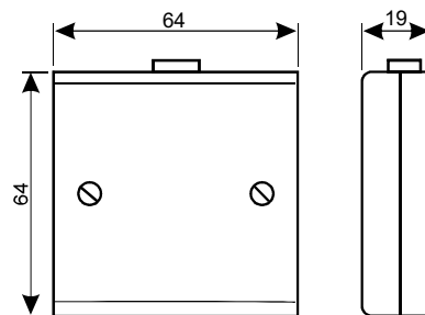
Габаритные размеры конвертера Z-397 (мод. USB Guard)
