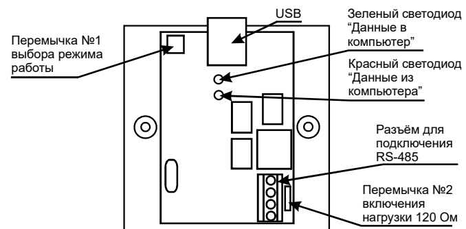
Расположение элементов на плате конвертера
