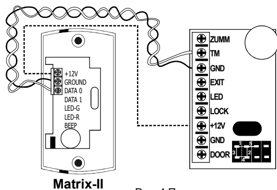
Рис. 4 Подключение внешнего считывателя
