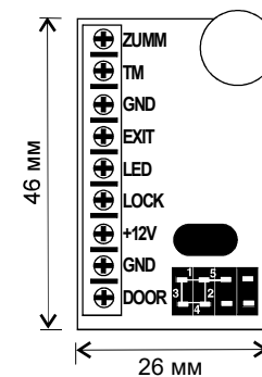
Рис.2 Внешний вид платы
