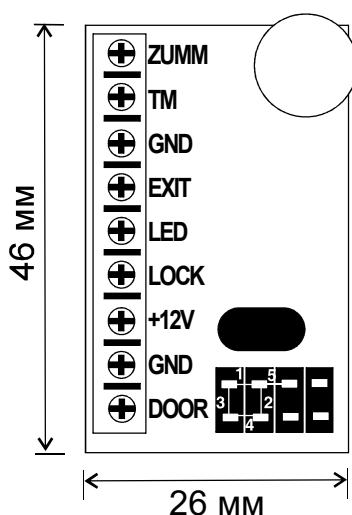
Рис.2 Внешний вид платы контроллера
