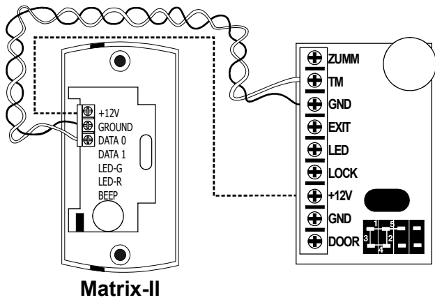
Рис. 4 Подключение внешнего считывателя
