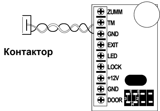
Рис. 5 Подключение контактора
