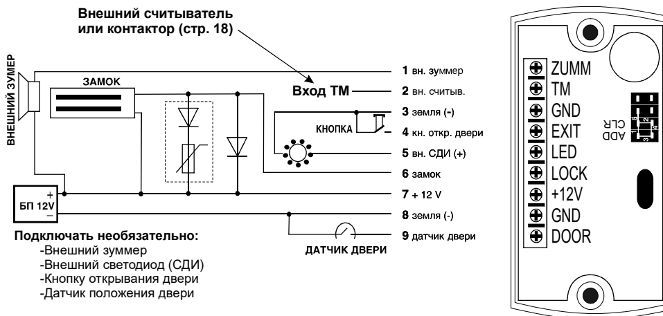
Рис. 6 Подключение внешних устройств
