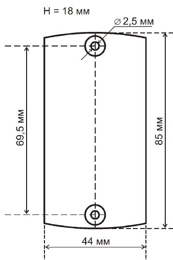
Рис.1 Габаритные размеры контроллера
