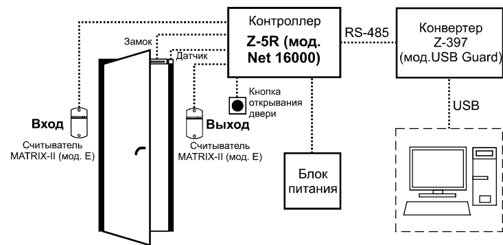
Рис.1 Схема СКУД с контроллером Z-5R (мод. Net 16000)
