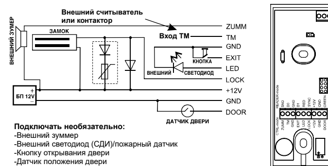
Рис.8 Подключение внешних устройств к контроллеру.
