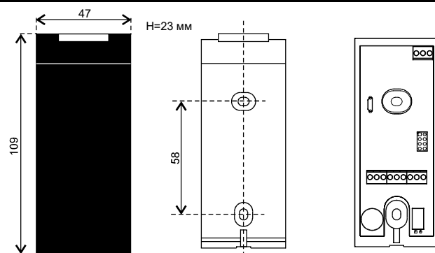
Рис.7 Габариты и монтажные отверстия.
