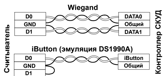
Рис.4 Схема подключения к контроллеру.
