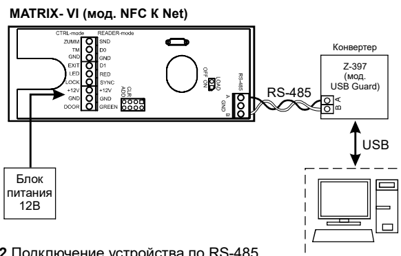
Рис.2 Подключение устройства по RS-485.
