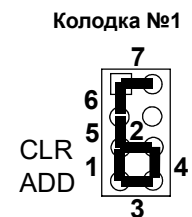
Рис.5 Положения переключателя.
