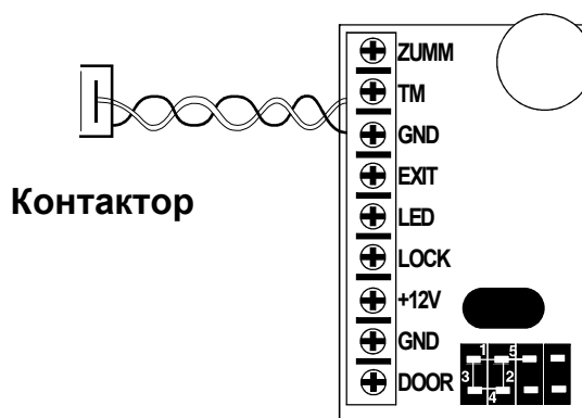
Рис. 5 Подключение контактора
