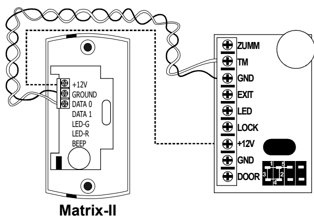
Рис. 4 Подключение внешнего считывателя
