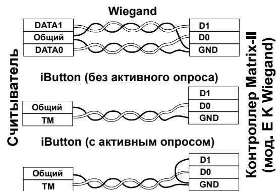
Рис.4 Варианты подключения Внешних считывателей
