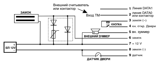
Рис.5 Схема подключения внешних устройств
