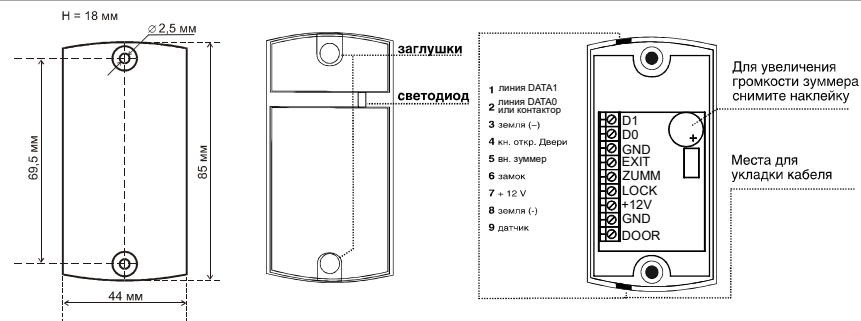
Рис.1 Габаритные размеры контроллера
