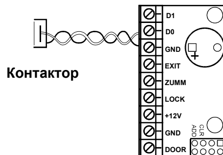
Рис. 4 Подключение контактора
