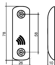
Рис.1 Габариты изделия.
